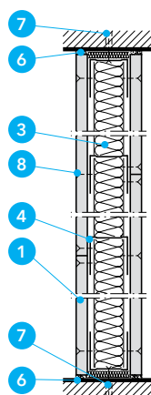
Przekrój A-A Detal B - Pionowy przekrój dla ściany EI 90
