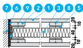
Przekrój B-B dla ściany EI 120 Detal C - Przekrój poprzeczny ściany
