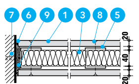
Przekrój B-B dla ściany EI 90
